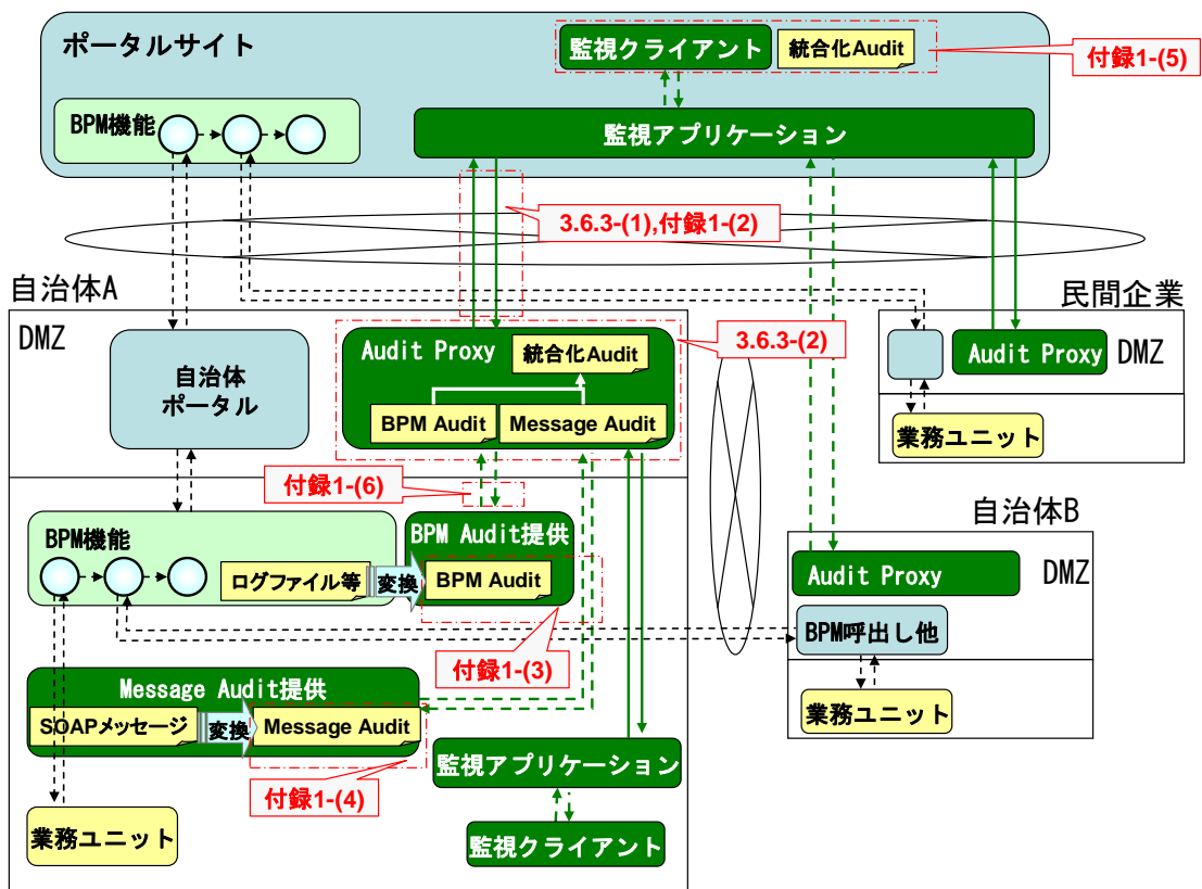
図3.6.1 モニタリング機能の実装模式図
