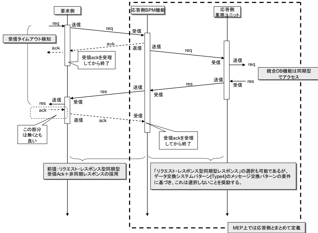
図3. 8. 14 リクエスト・レスポンス型同期型受信Ack+非同期型レスポンスの組み合わせ制約(奨励しない)
