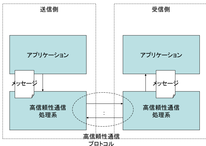
図 3. 1. 6 高信頼性通信機能
