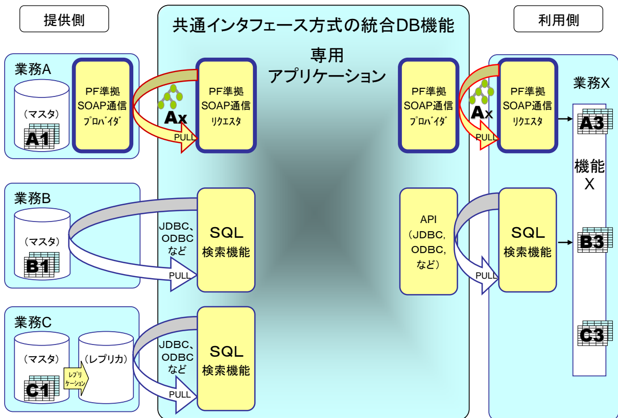
図3. 2. 22は、専用のアプリケーションによる実装パターンである。
