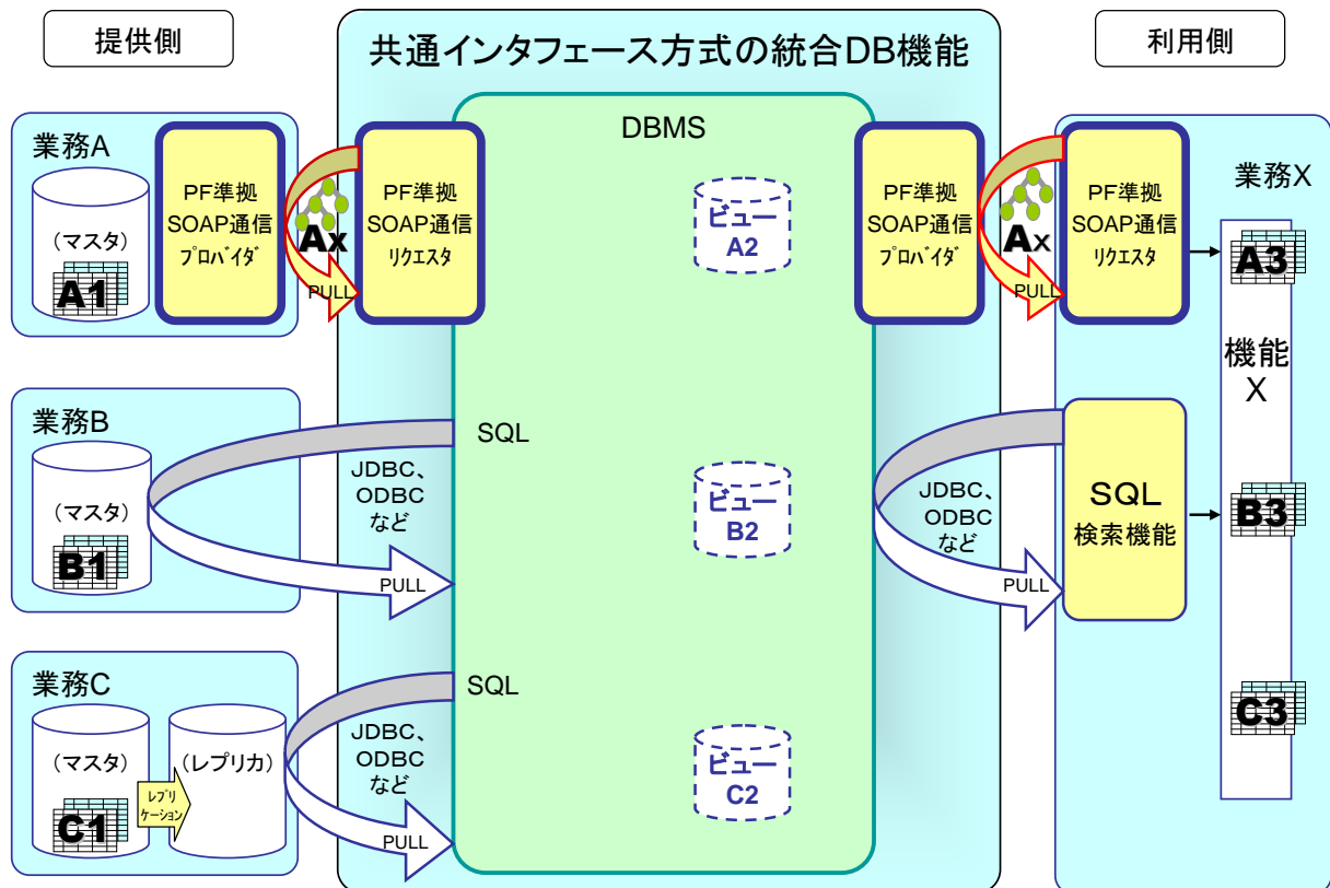
図 3. 2. 20 共通インターフェース方式の統合 DB 実装パターン(1)
