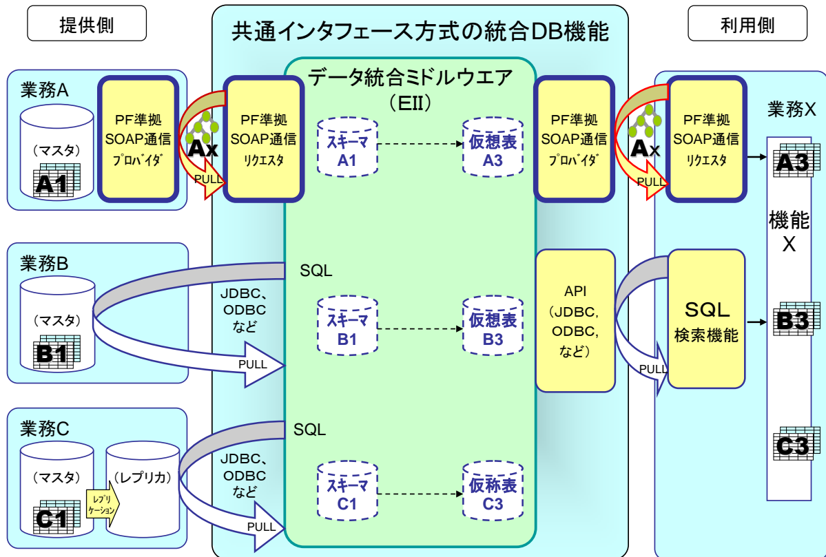
図3. 2. 21 共通インターフェース方式の統合 DB 実装パターン(2)
