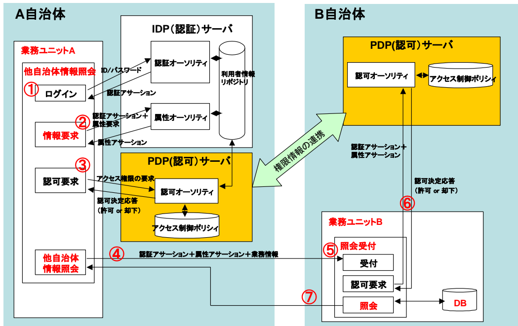
図3. 5. 2.3 権限管理基盤技術のユースケース
