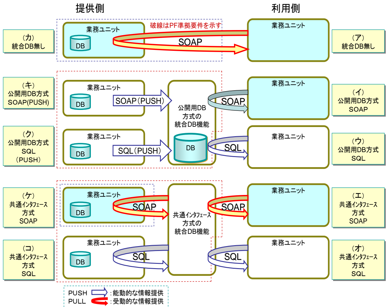
図3. 2. 16 統合DB機能の方式とインターフェースのまとめ
