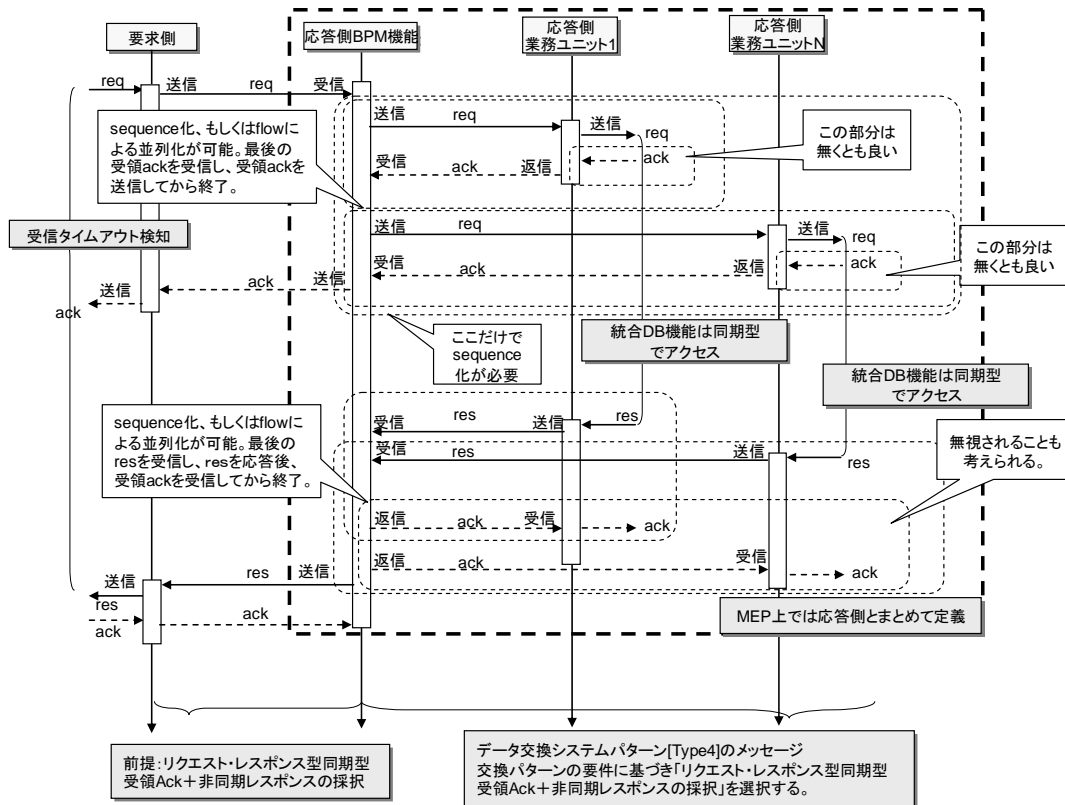
図3. 8. 13 リクエスト・レスポンス型同期型受領 Ack+非同期型レスポンスの組み合わせ制約(一般的な構成)
