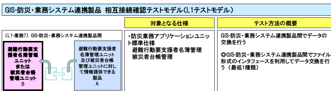
図8 地域情報 PF 相互接続確認テストモデル (L1 テストモデル) (4/4)
