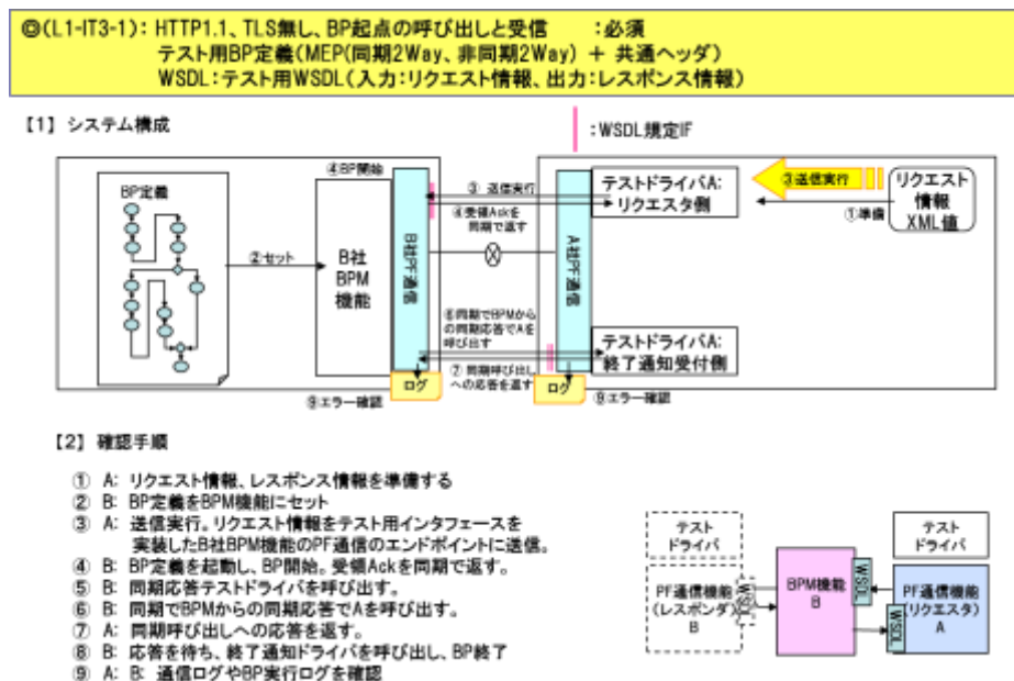
図 1 5 BPM 機能： L1 テストモデルの確認環境と確認手順（（L1-IT3-1））
