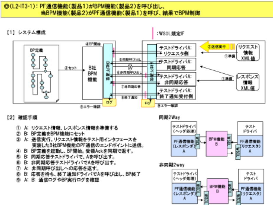
図 2 4 BPM 機能：3 社モデル：L2 テストモデルの確認環境と確認手順（(L2-IT3-1)）
