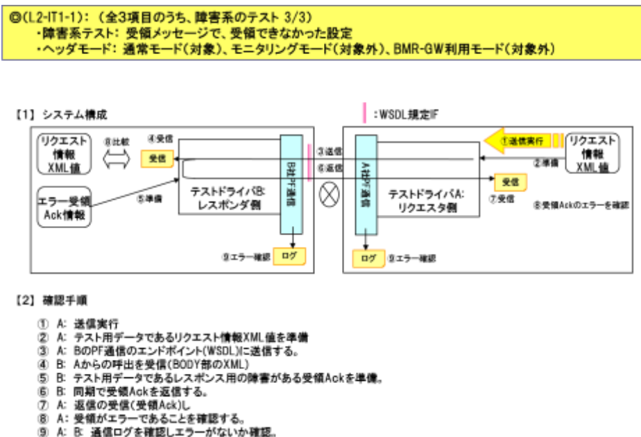
図 2 3 PF 通信機能： L2 テストモデルの確認環境と確認手順 ( (L2-IT1-1 (障害系テスト)) )
