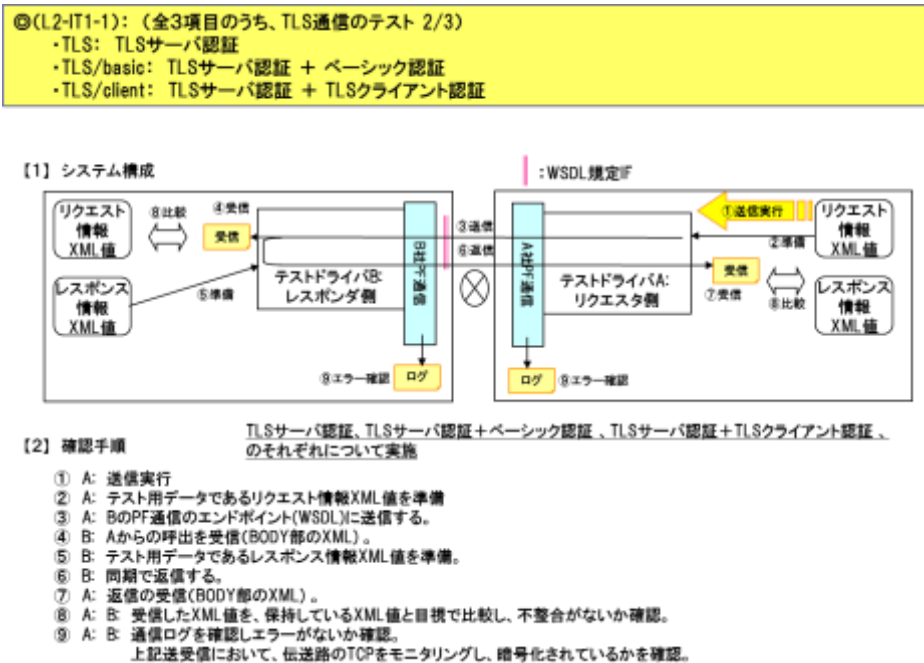
図 2 2 PF 通信機能： L2 テストモデルの確認環境と確認手順 ( (L2-IT1-1 (TLS 通信)) )
