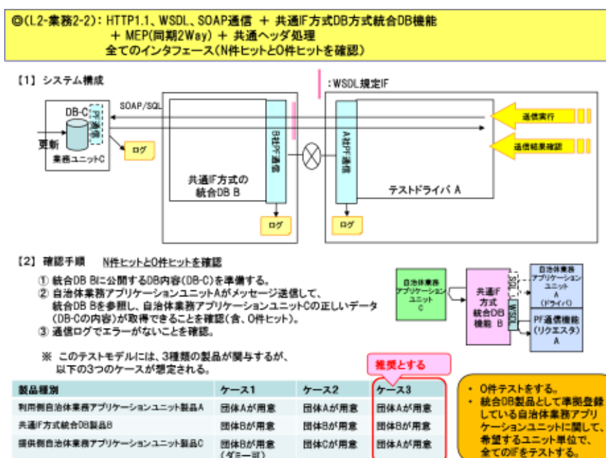
図 2 7 共通 IF 方式統合 DB 機能 : L2 テストモデルの確認環境と確認手順 ( (L2-業務 2-2) )
