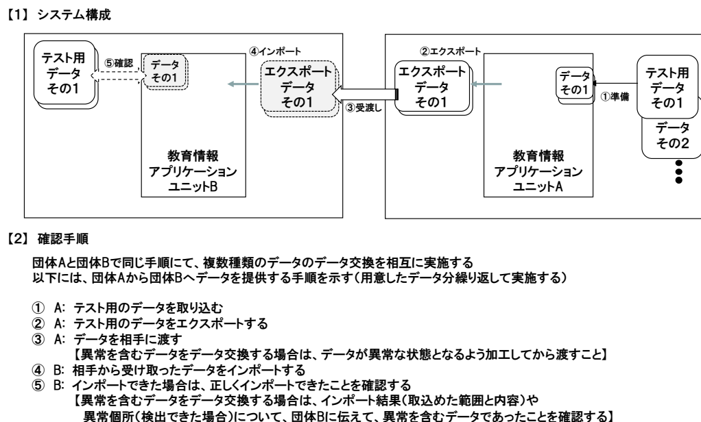
図 2 9 教育情報アプリケーションユニット: L2 テストモデルの確認環境と確認手順 ( (L2-業務 5) )
