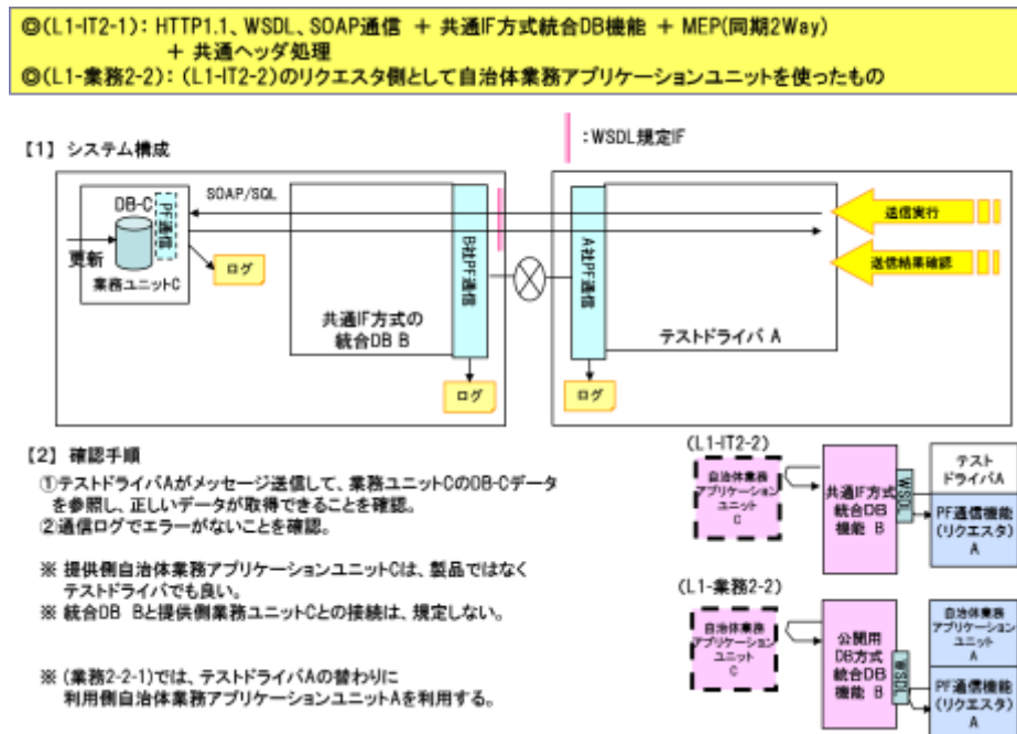
図 1 4 共通 IF 方式統合 DB 機能： L1 テストモデルの確認環境と確認手順（（L1-IT2-2）（L1-業務 2-2））
