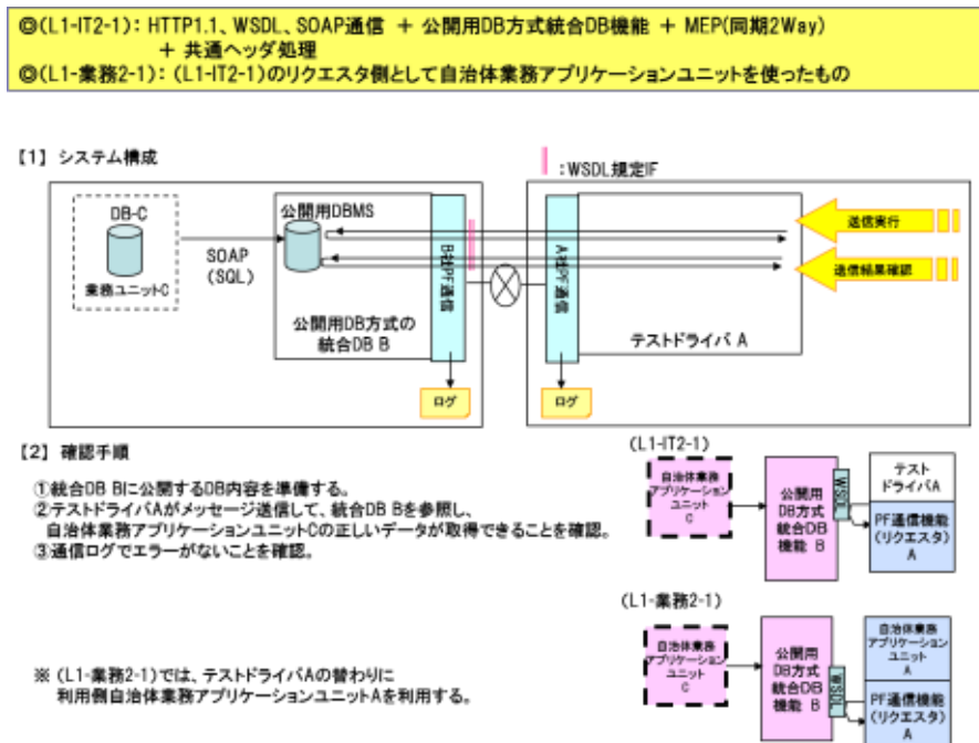
図 1 3 公開用 DB 方式統合 DB 機能： L1 テストモデルの確認環境と確認手順 （（L1-IT2-1）（L1-業務 2-1））
