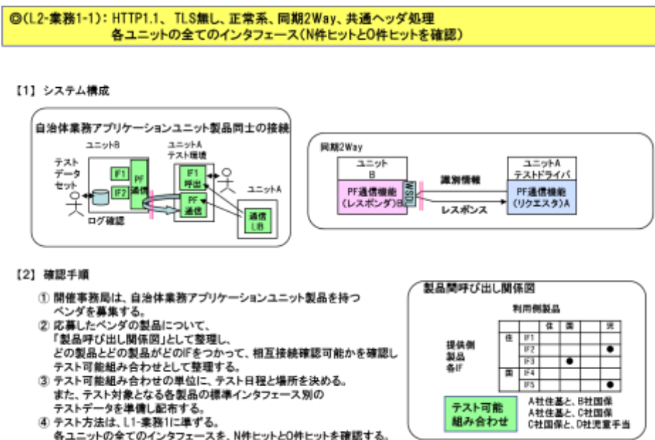
図 2 5 業務ユニット：全インタフェース：L2 テストモデルの確認環境と確認手順 ( (L2-業務 1-1) )
