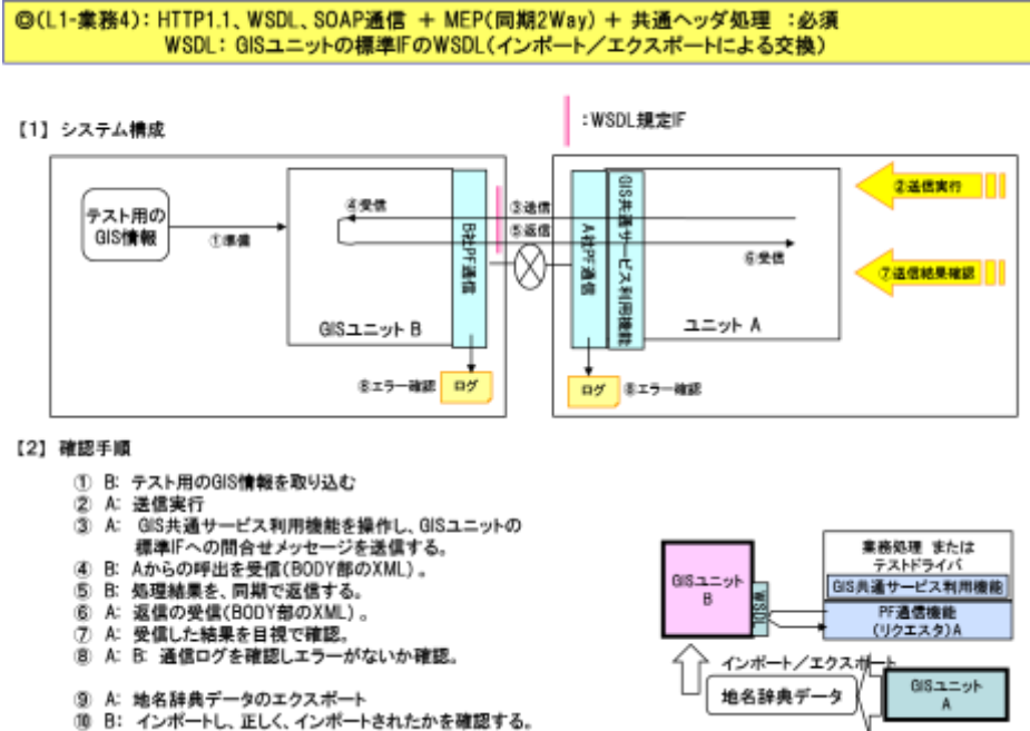
図 1 8 GIS ユニット： L1 テストモデルの確認環境と確認手順（（L1-業務4））
