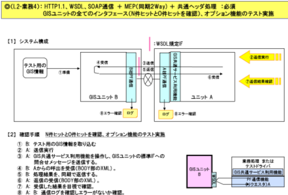
図 2 8 GIS ユニット:オプション: L2 テストモデルの確認環境と確認手順 ( (L2-業務 4-2) )
