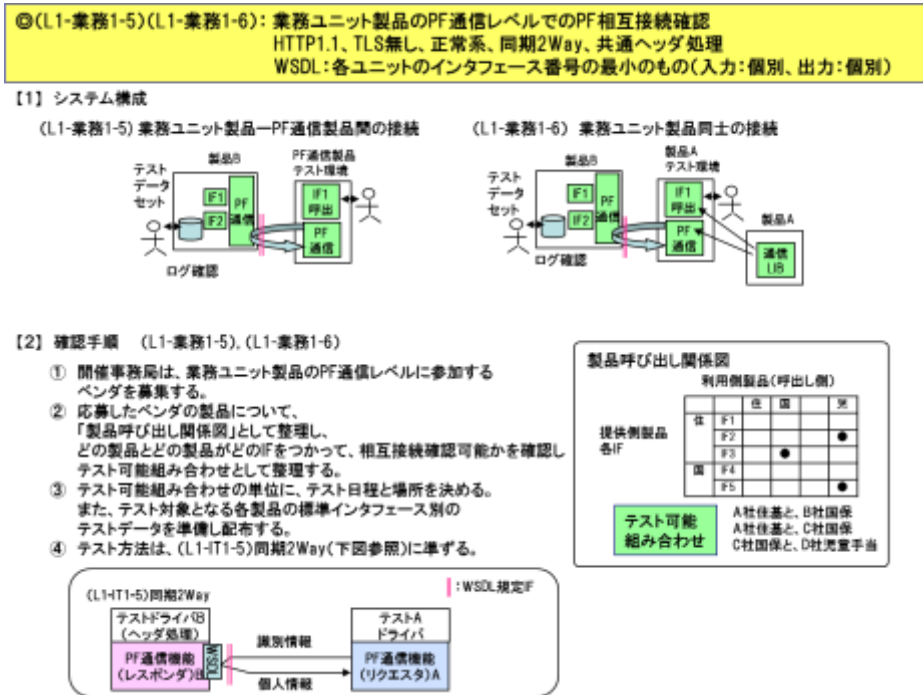
図 1 6 ユニットと PF 通信機能 : L1 テストモデルの確認環境と確認手順 ( (L1-業務 1-5) (L1-業務 1-6) )
