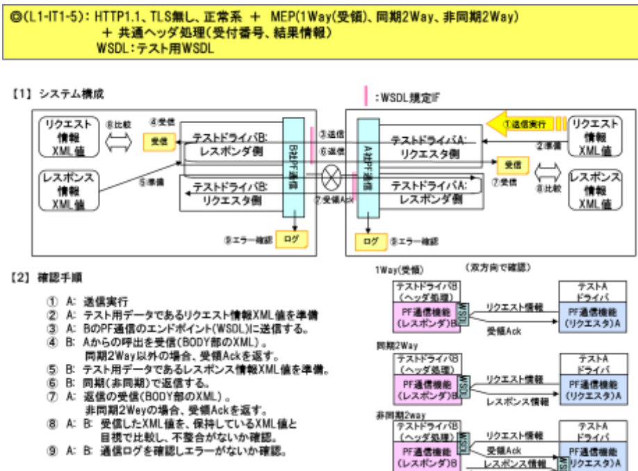
図 1 2 PF 通信機能： L1 テストモデルの確認環境と確認手順（（L1-IT1-5））
