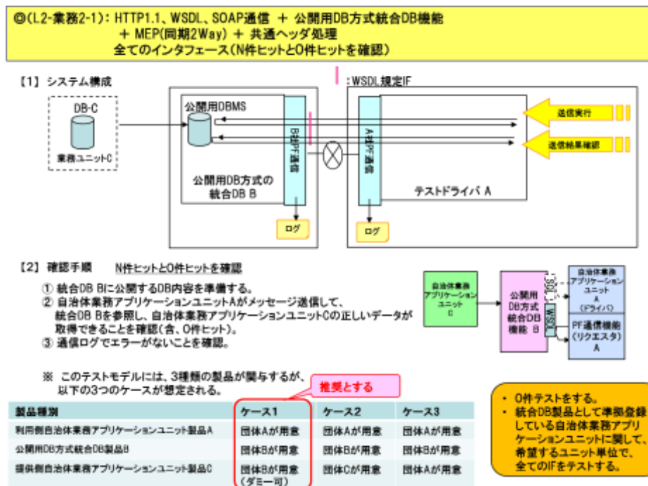
図 2 6 公開用 DB 方式統合 DB 機能 : L2 テストモデルの確認環境と確認手順 ( (L2-業務 2-1) )
