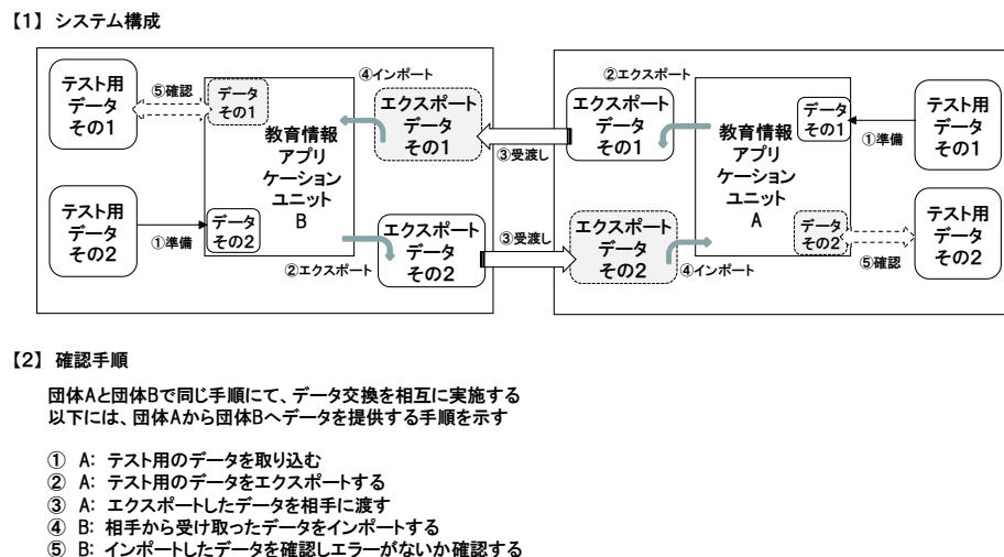
図 1 9 教育情報アプリケーションユニット： L1 テストモデルの確認環境と確認手順 （（L1-業務5））
