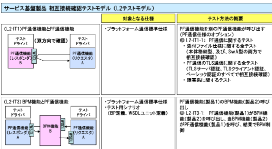
図9 地域情報 PF 相互接続確認テストモデル (L2 テストモデル) (1/3)
