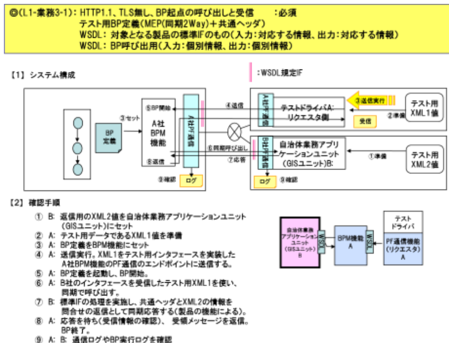
図 1 7 BPM 機能 : L1 テストモデルの確認環境と確認手順 ( (L1-業務 3-1) )
