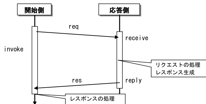
図 4. 4 リクエスト・レスポンス型同期型レスポンス
